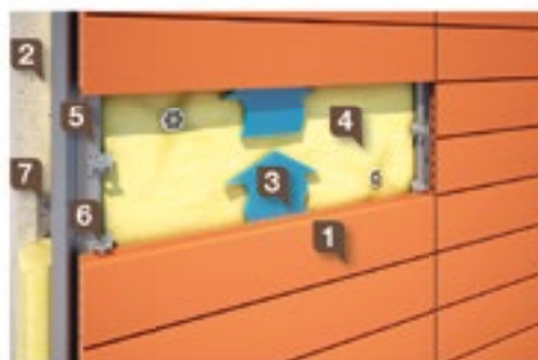
Pherak® Slim con struttura a montanti verticali e clips
