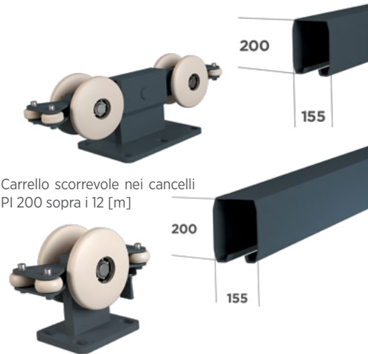
Carrello scorrevole nei cancelli PI 200 sopra i 12 [m]
