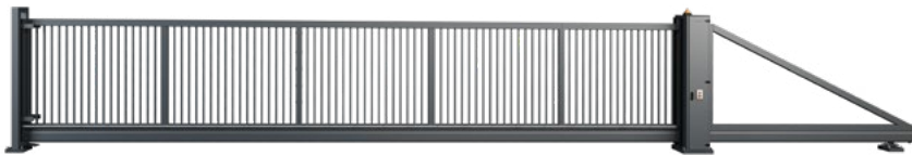
Riempimento in tubo tondo 25 [mm] (saldato alla struttura)
