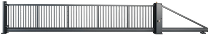
Riempimento in profilati 30x18 [mm] (saldato alla struttura)
