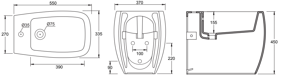
33110101 BIDET NUR Bidet monoforo Bidet Nur single tap hole
