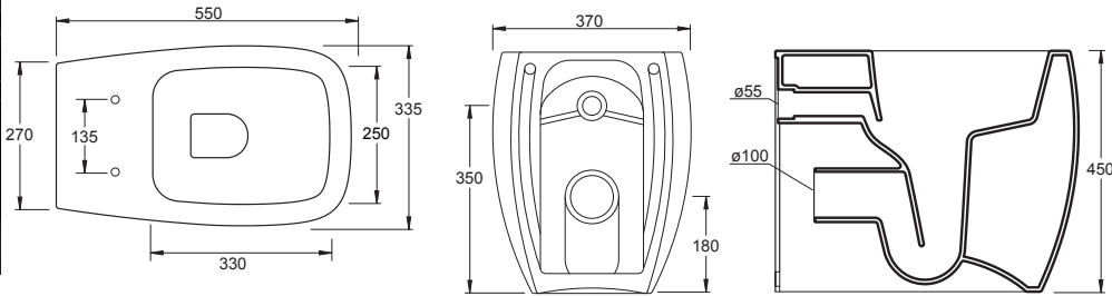
33110101 BIDET NUR Bidet monoforo Bidet Nur single tap hole
