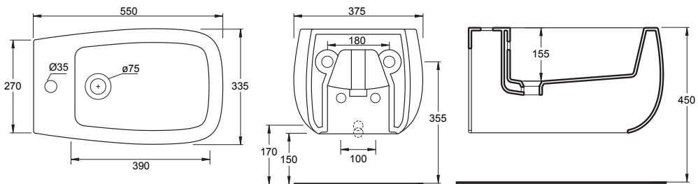
33130101 BIDET NUR sospeso Bidet sospeso monoforo Bidet Nur wall hung single tap hole
