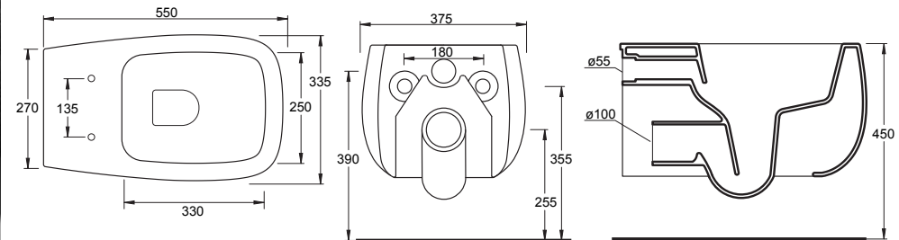
33120101 VASO NUR SOSPESO Vaso sospeso Nur Wc wall hung Nur
