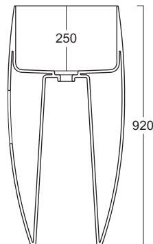
33230101 Lavabo freestanding NUR OPEN 33230101 Washbasin freestanding NUR OPEN
