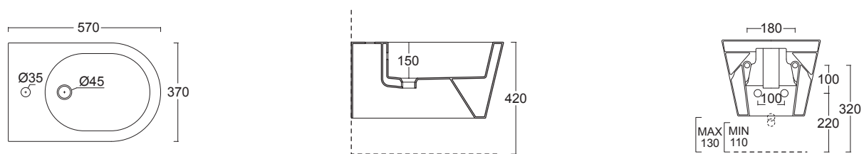
31180101 Bidet sospeso HIDE ROUND 31180101 Wall hung bidet HIDE ROUND
