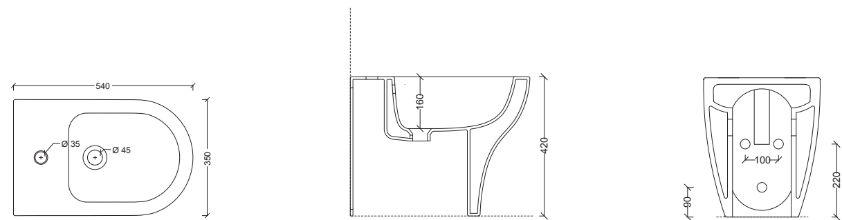
32210101 Bidet UNICA
