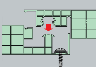
Particolare di aggancio lastre
