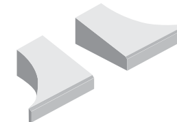
Coppia Terminali scivolo passo carraio Disponibile nei colori grigio e testa di moro. Vendibile solo a coppie. Couple of driveway terminal slide Available in grey and dark brown colour saleble only in couples. Dimensioni - Dimensions 400 X h 450 mm
