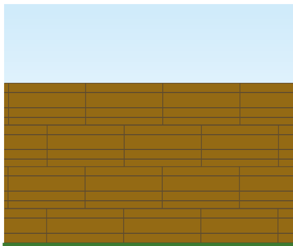
MURO CHIUSO pezzi mq. nr. 26,5 - peso per mq. 690.
