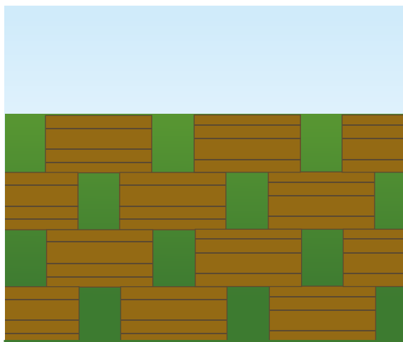
MURO APERTO pezzi mq. nr. 18,5 - peso per mq. 481.
