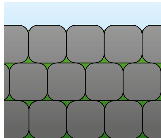
MURO ALTERNATO A SCARPATA. ESCAPMENT ALTERNATE WALL
